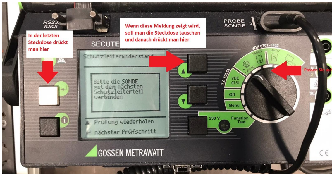
Bild 6.: Meldung um die Steckdose zu tauschen
